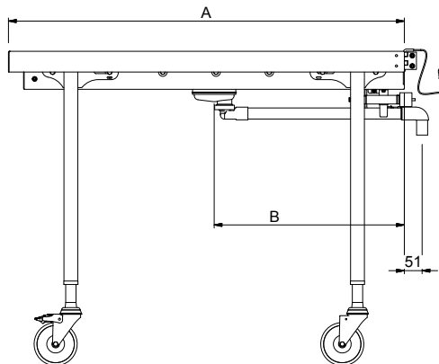
Front aanzicht
